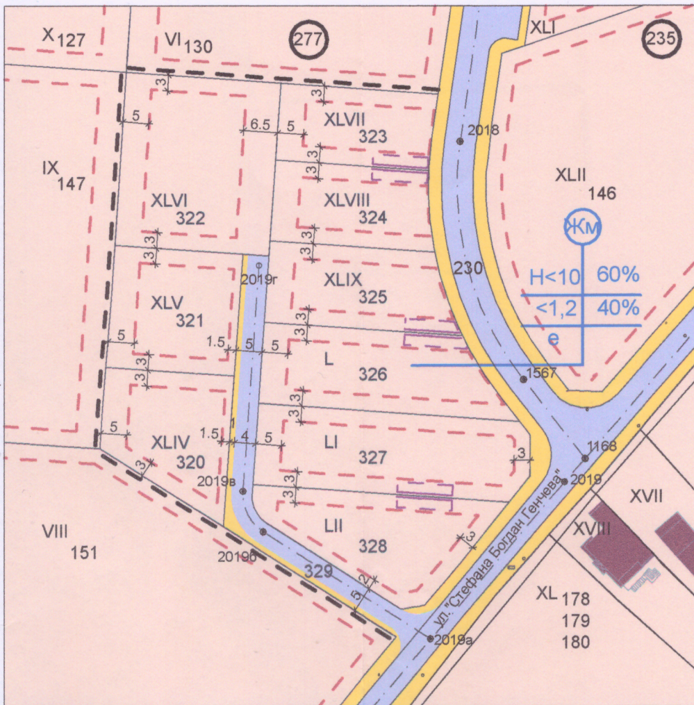
ПРОЕКТ ЗА ЧАСТИЧНО ИЗМЕНЕНИЕ НА ПОДРОБЕН УСТРОЙСТВЕН ПЛАН -ПЛАН ЗА ЗАСТРОЯВАНЕ, М 1:1000
