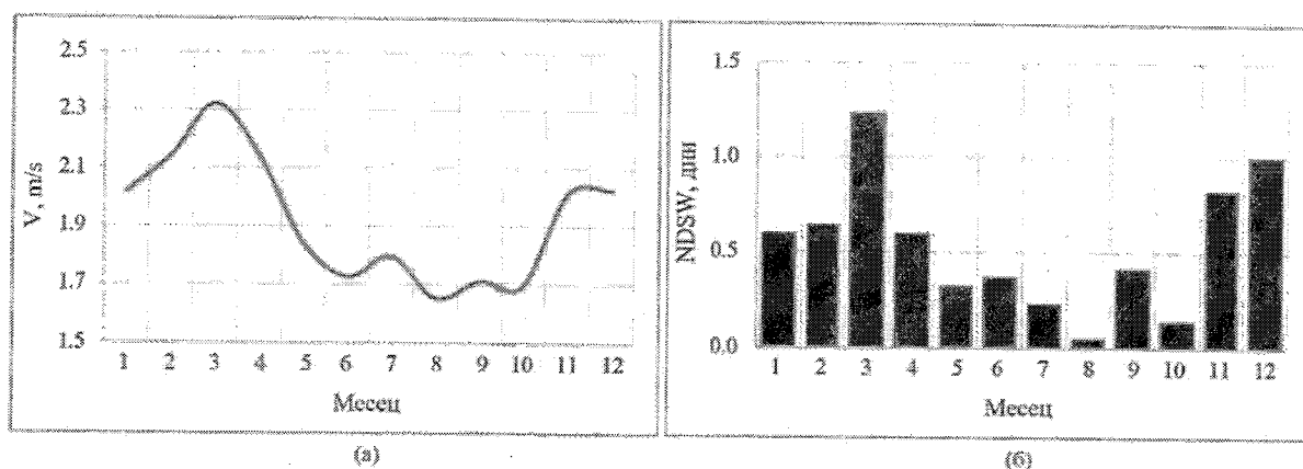
Фигура 8. Годишен ход на: (а) средната скорост на вятъра ( V , m/s) и (б) брой дни със силен вятър (NDSW) в метеорологична станция Габрово за периода 2001 – 2022 г. (Източник: НИМХ)
